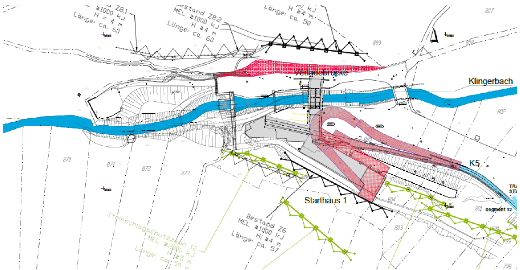
LAGEPLANAUSZUG BEREICH STARTHAUS 1 M. 1:500
